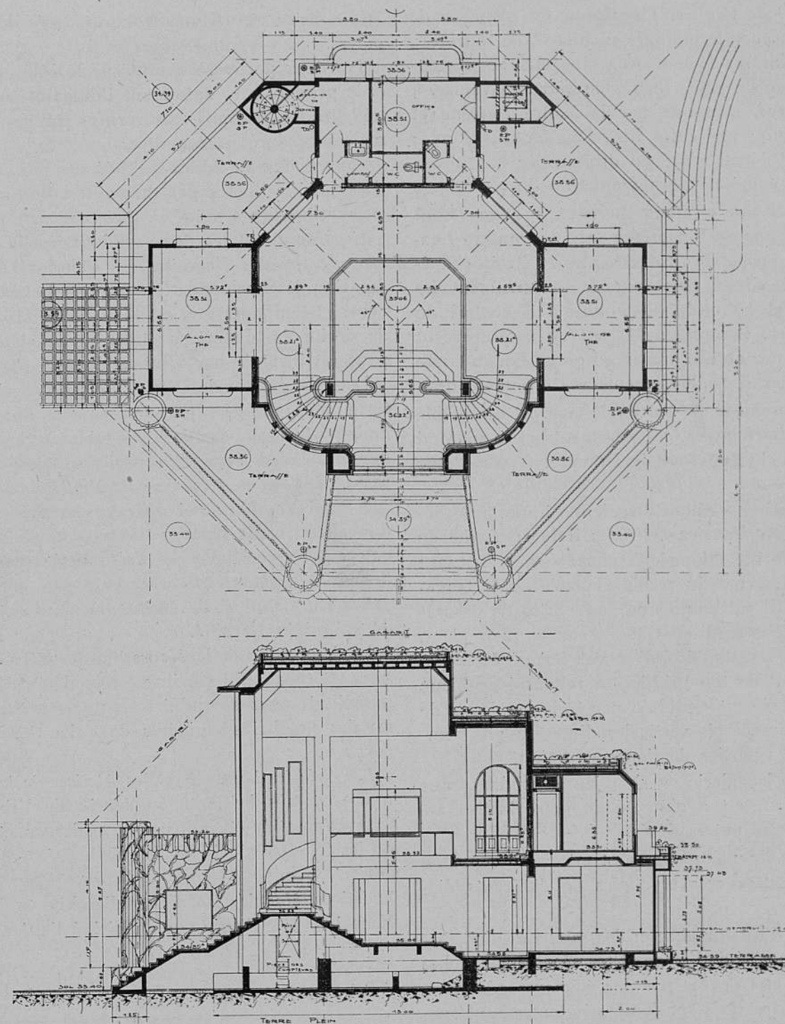
Pavillon des Galeries Lafayette. — Étage et Coupe. — Architectes : MM. HIRIART, TRIBOUT ET BEAU.
