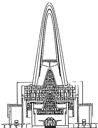
André Dunoyer de Segonzac. Basilique de la Altagracia à Higüey, République Dominicaine: perspective de la façade ouest (1949)
